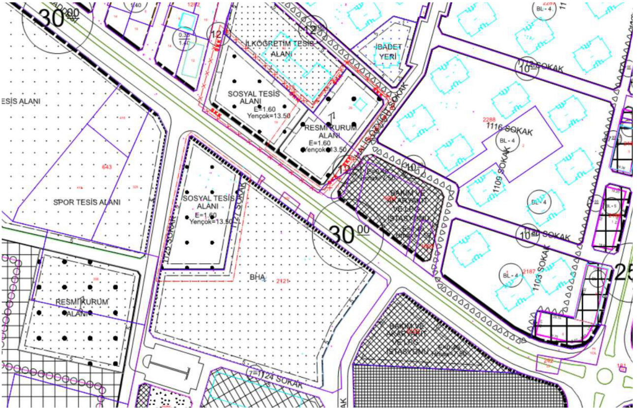
1/1000 ÖLÇEKLİ ÖNERİ UYGULAMA İMAR PLANI
